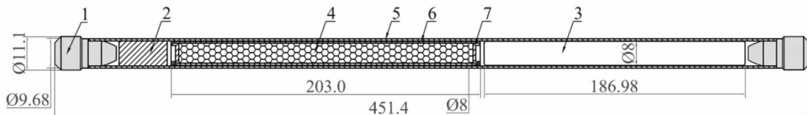
1. 外端塞；2. 垫块；3. 钴棒；4. 源芯；5. 外包壳；6. GYB型源包壳 RSCOGYB 型特殊形式放射性物品结构示意图
