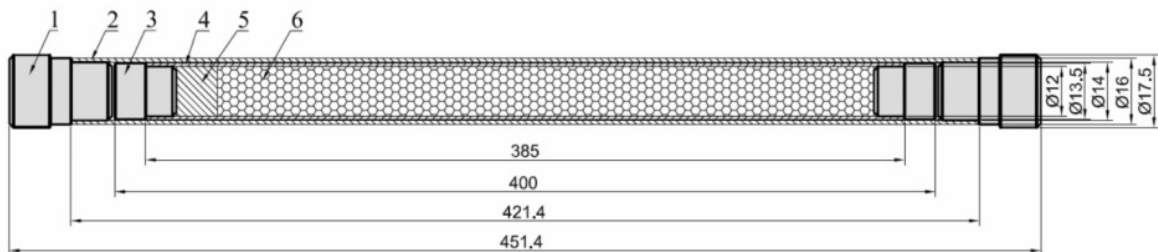
1. 外端塞；2. 外包壳；3. 内端塞；4. 内包壳；5. 垫块；6. 源芯 RSCOGYZLY 型特殊形式放射性物品结构示意图
